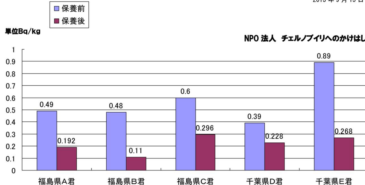
2013年 保養前・後の尿放射能分析結果（セシウム 134 + セシウム 137）
